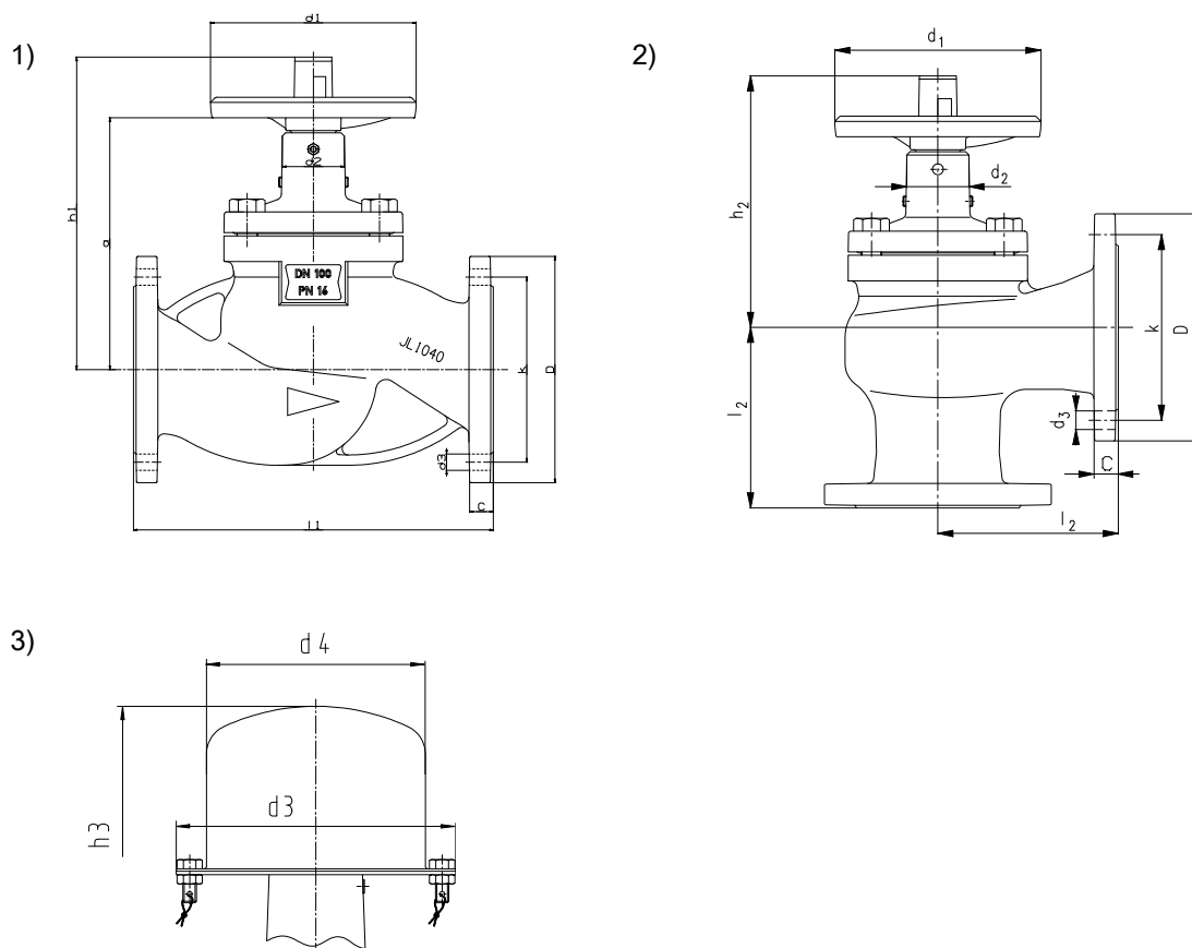
Рис. 3: 1) Проходная арматура; 2) Угловая арматура; 3) Пломбируемая крышка-колпак для предотвращения несанкционированного срабатывания, монтажный комплект
