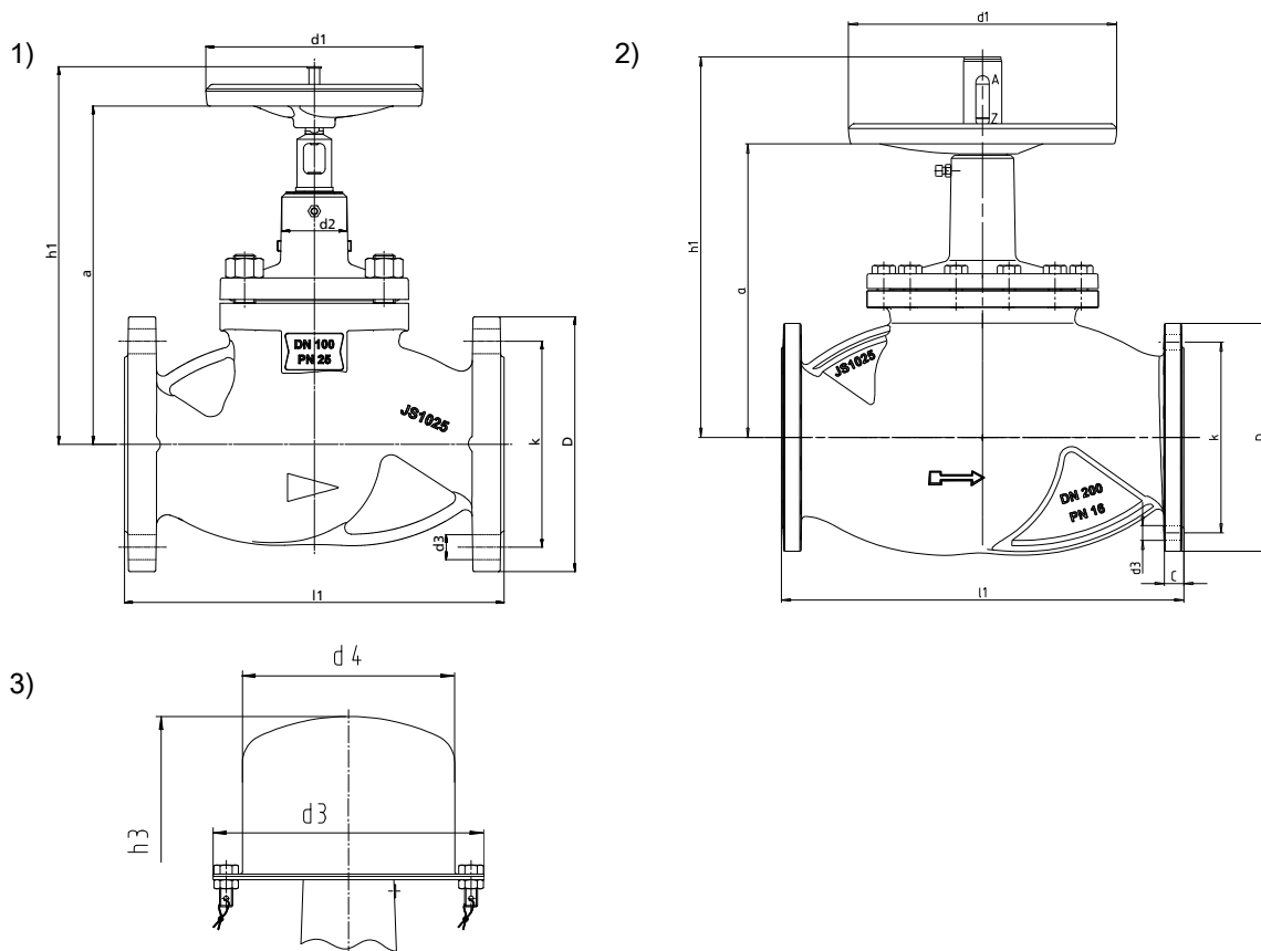
Рис. 4: 1) PN 16/25 до DN 150; 2) PN 16 DN 200–350; 3) Пломбируемая крышка-колпак для предотвращения несанкционированного срабатывания, монтажный комплект
