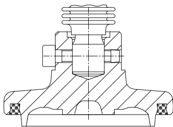
Редукционный золотник с уплотнительным кольцом из ПТФЭ, DN 15 - 100
